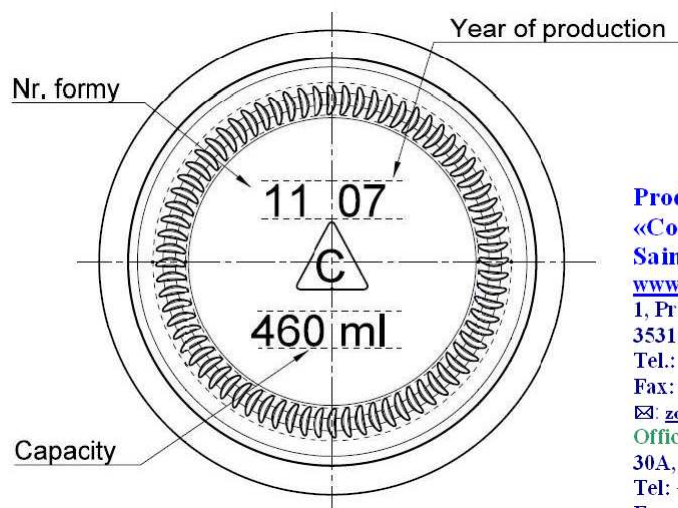
Bottom view Scale: 1:1
